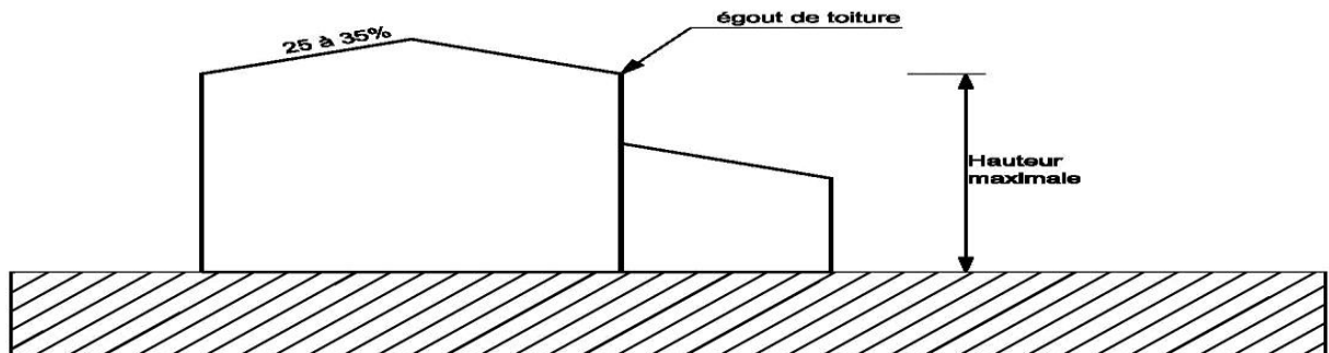
cas d'une construction avec une toiture à plusieurs pentes
